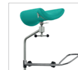
Упоры для стоп WF-23.0, установленные на кронштейне подколенника
